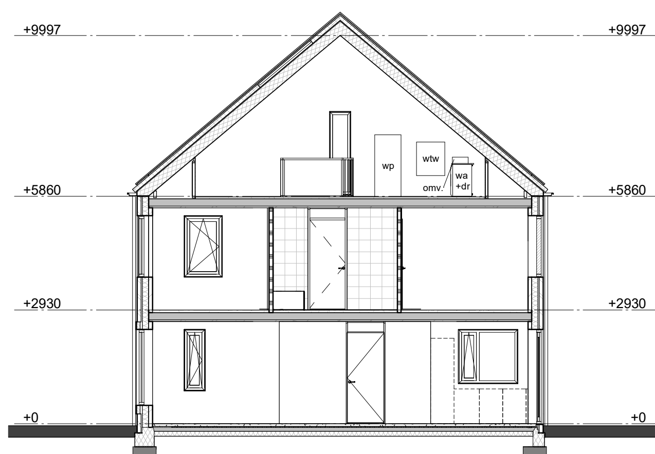
DOORSNEDE C-A
