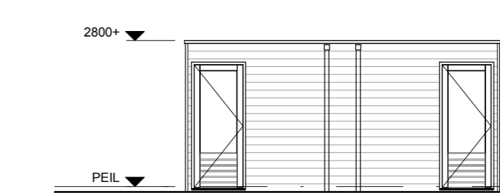
VOORGEVEL BERGING
