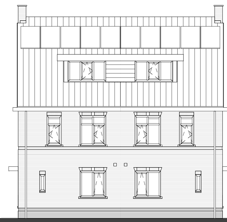
WC01 VOORGEVEL
