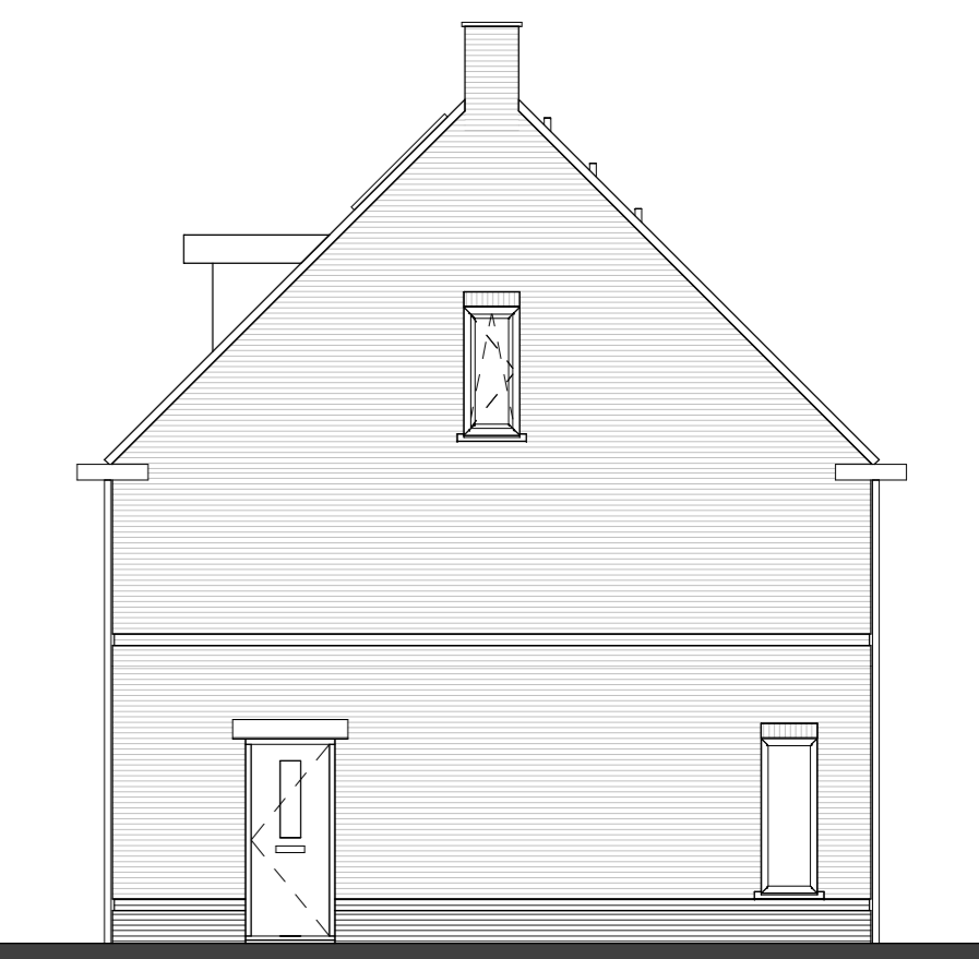
RECHTERGEVEL
