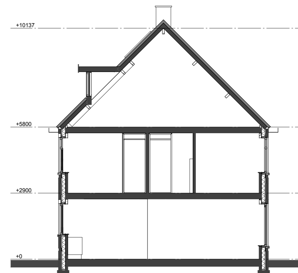
PRINCIPE DOORSNEDE B
