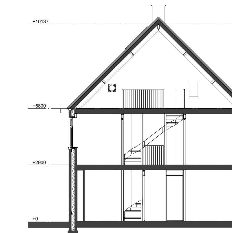
PRINCIPE DOORSNEDE A
